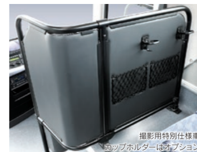
運転席仕切(標準パイプタイプ)
